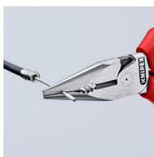
Gefräste Nut im Greifbereich
