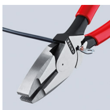
09 11/12 240: Universelle Dorn-Crimpstelle unterhalb des Gelenks
