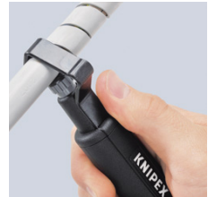
Wendelschnitt
