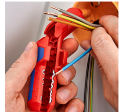
Abisolieren von Einzelleitern
