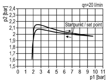
Hysteresese
