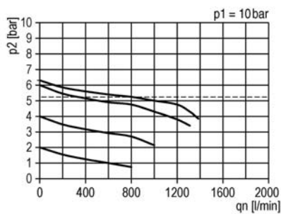
Durchflussdiagramm
