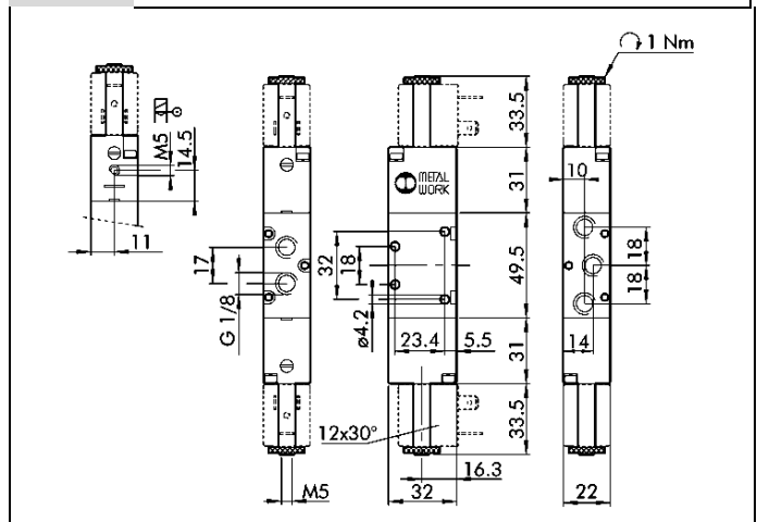
5/2 Bistabil mit ohne Differenzialkolben G 1/8
