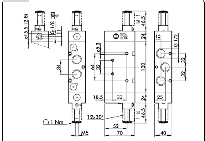
5/2 Bistabil mit ohne Differenzialkolben G 1/2
