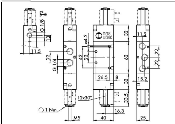
5/2 Bistabil mit ohne Differenzialkolben G 1/4
