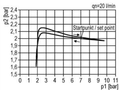
Hysteresese
