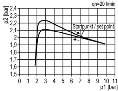
Hysterese
