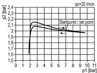
Hysterese
