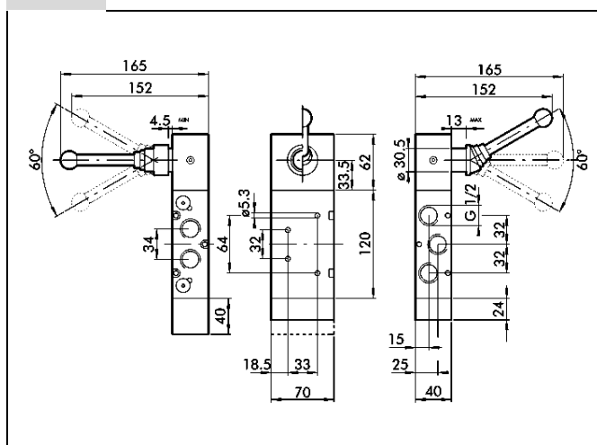
5/3 90°-Hebel G 1/2
