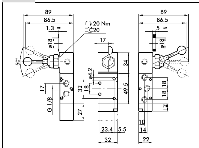
5/3 90°-Hebel G 1/8
