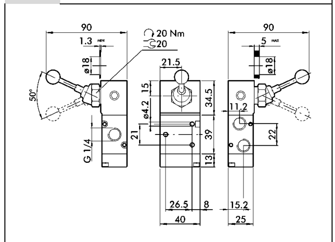
3/2 90°-Hebel G 1/4
