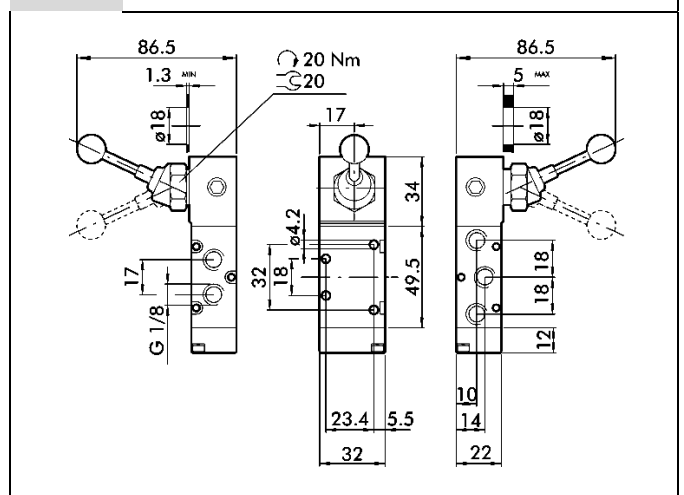
5/2 90°-Hebel G 1/8
