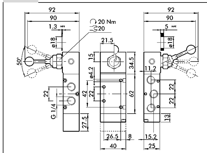
5/3 90°-Hebel G 1/4
