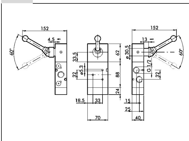
3/2 90°-Hebel G 1/2
