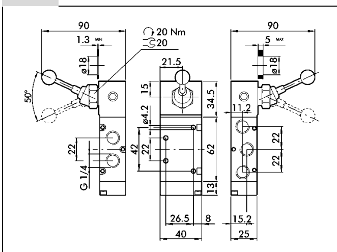
5/2 90°-Hebel G 1/4
