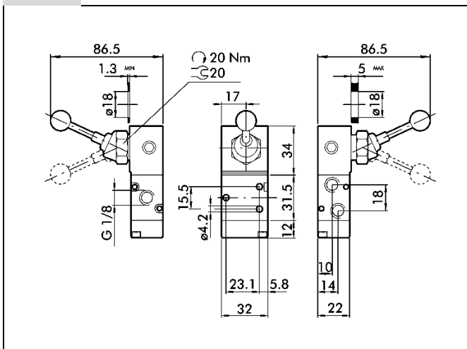
3/2 90°-Hebel G 1/8
