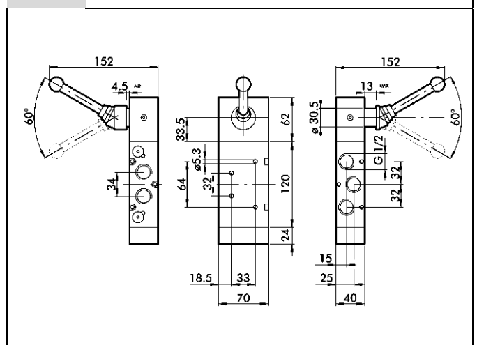
5/2 90°-Hebel G 1/2
