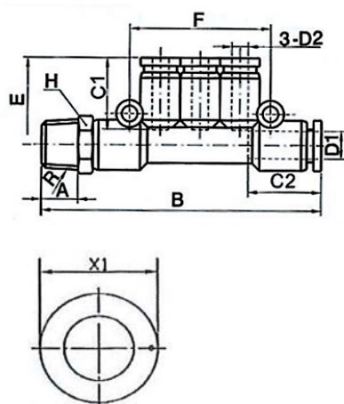
Verteiler-Steckverschraubung , drehbar, konisches Aussengewinde nach ISO 7-1
