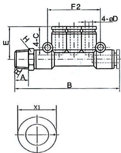
Verteiler-Steckverschraubung , drehbar, konisches Aussengewinde nach ISO 7-1
