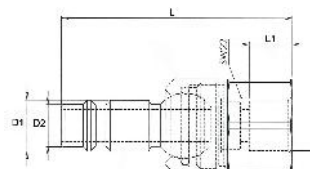
Nippel, drehbar
