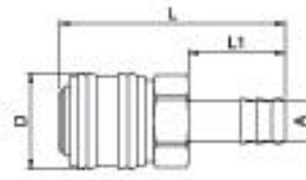
Schlauchtülle
