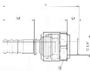
Schlauchtülle, Außengewinde
