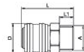
Außengewinde
