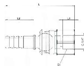
Schlauchtülle, Innengewinde
