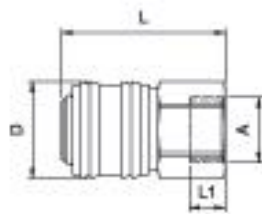
Innengewinde
