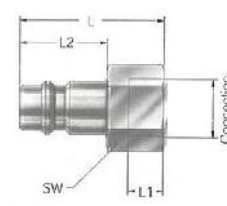
Nippel mit Innengewinde
