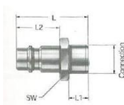
Nippel mit Außengewinde
