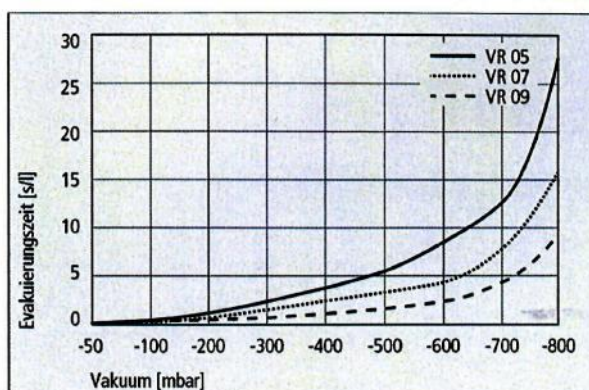
Evakuierungszeit für unterschiedliche Vakuum-Bereiche
