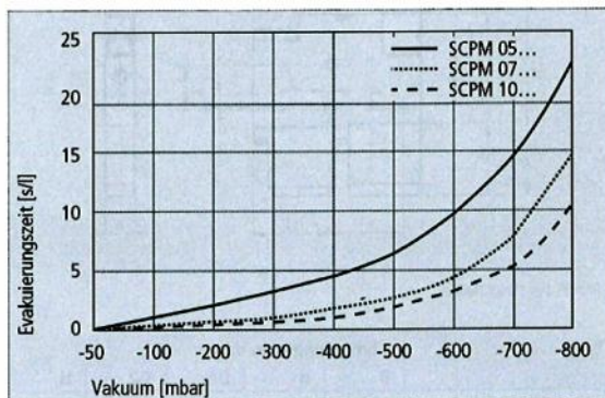
Evakuierungszeit für unterschiedliche Vakuumbereiche
