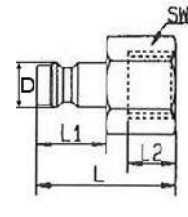
Nippel (Innengewinde)
