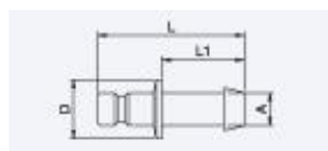
Tülle
