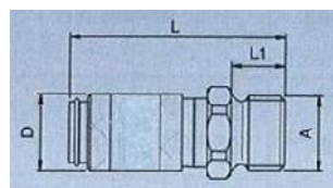
Außengewinde
