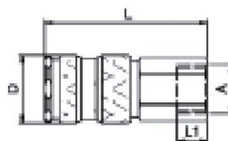
Innengewinde
