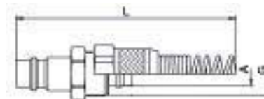
Nippel für Schlauch mit Überwurfmutter, Knickschutzfeder
