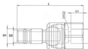
Nippel, drehbar
