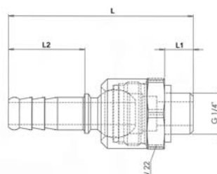
Schlauchtülle, Außengewinde
