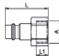
Nippel Innengewinde
