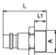
Nippel Außengewinde
