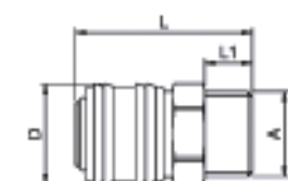
Außengewinde
