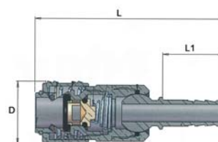
Schlauchtülle, drehbar
