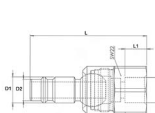
Nippel, drehbar
