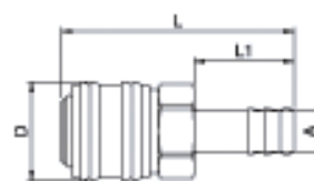
Schlauchtülle
