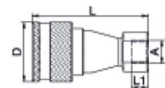
Kupplung
