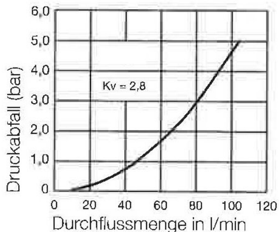
246.14 – G 1/2
