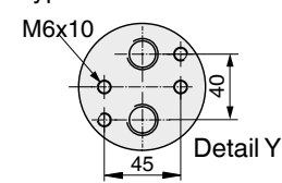
Typ 5000U
