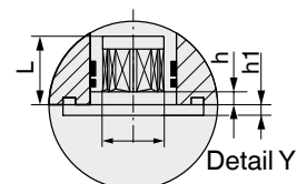
Typ 5000U
