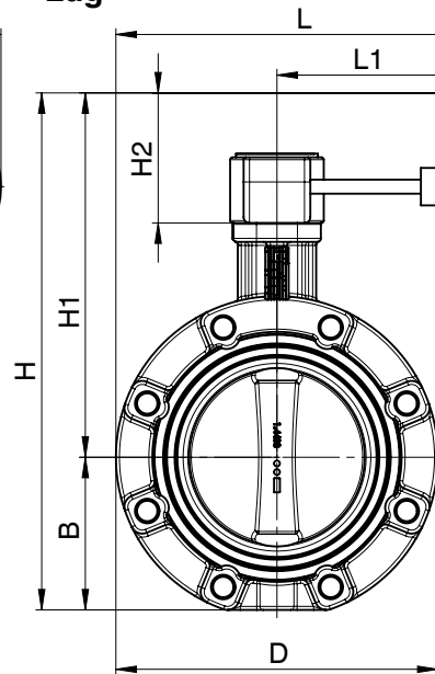
Lug
