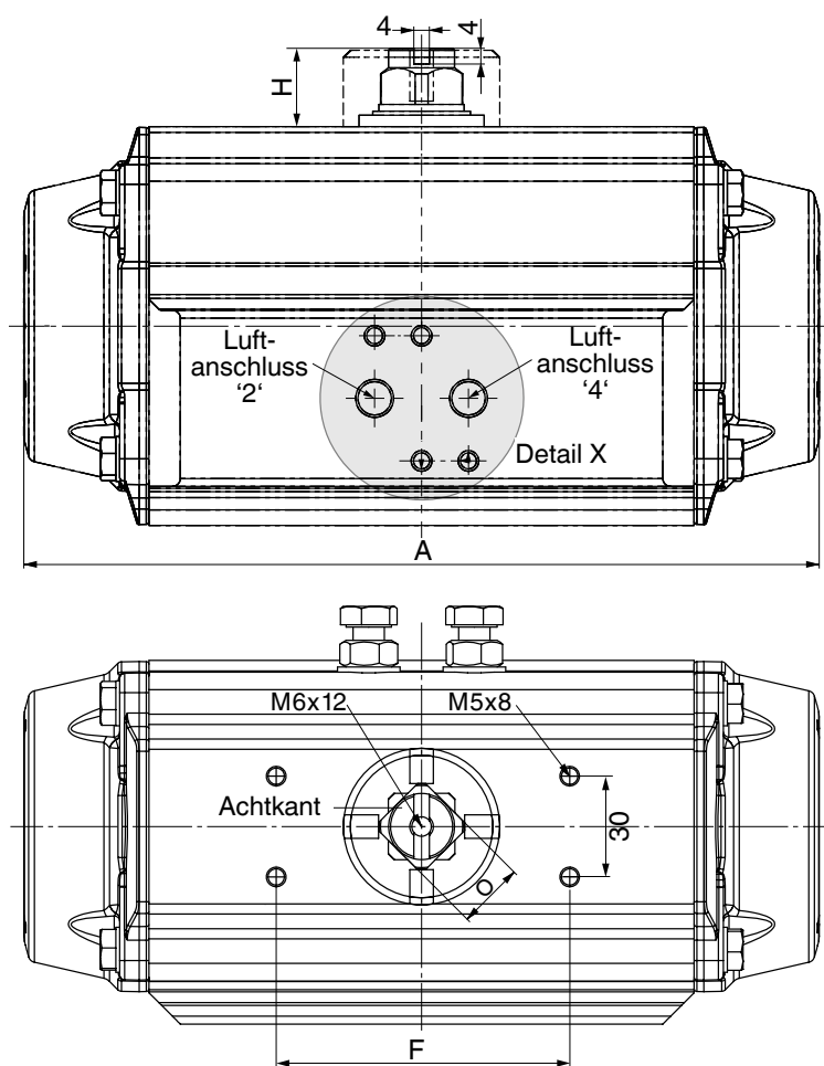
Typ 0015U-1200U
