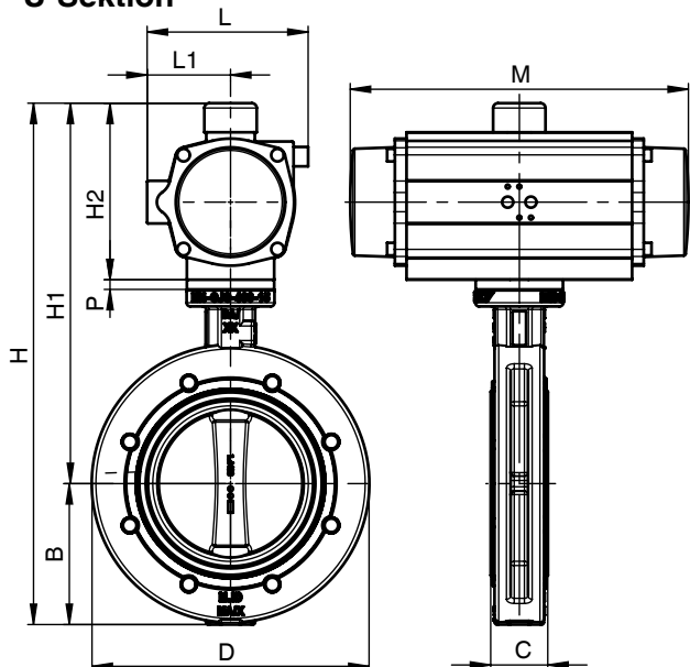
U-Sektion
