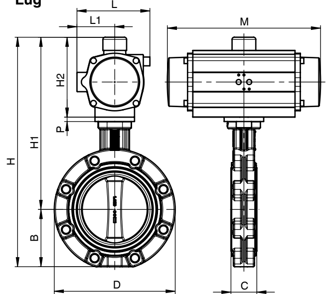
Lug
