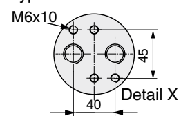
Typ 2000U-4000U
