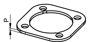
Distanzstück (DIS)
