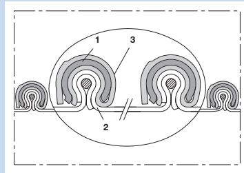
Abgasschlauch, vibrationsfest, äußeres Schutzprofil
