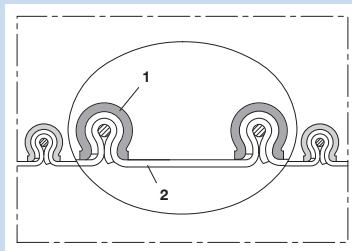
Hochtemperaturschlauch, Klemmprofilschlauch, (bis +400°C)
