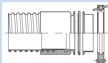
TRI-Clamp Kupplung passend zu Stutzen nach DIN 32676, lebensmittelecht
