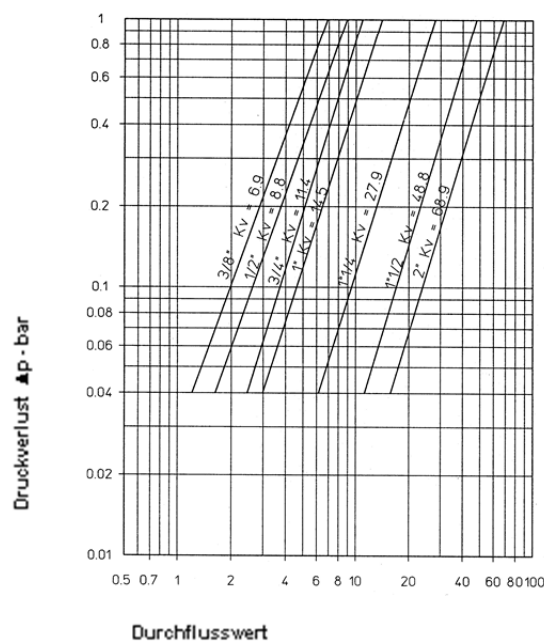
Durchfluss – Druckverlust Diagramm
