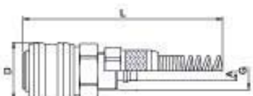
Schlauchanschluss, Überwurfmutter und Knickschutzfeder
