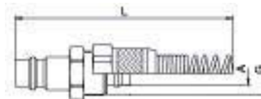
Nippel für Schlauch mit Überwurfmutter und Knickschutzfeder
