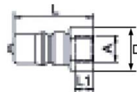
Nippel
