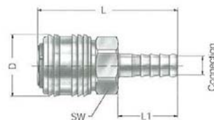
Schlauchanschluss
