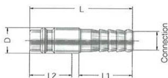
Tülle
