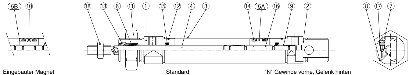
Eingebauter Magnet
