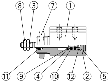
Eingebauter Magnetring
