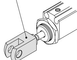
Montage des Gabelgelenks
