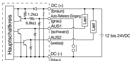
ZSE40 (F) ISE40-□-70 (L)-(M) mit Auto-Referenz-Eingang
