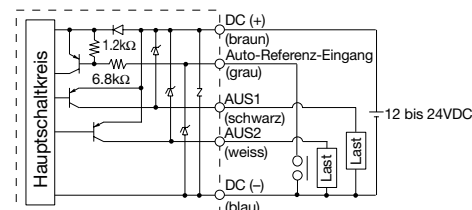
ZSE40 (F) ISE40-□-70 (L)-(M) mit Auto-Referenz-Eingang
