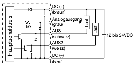
ZSE40 (F) ISE40-□-62 (L)-(M) mit Analogausgang
