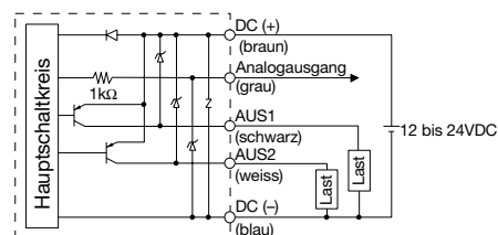
ZSE40 (F) ISE40-□-62 (L)-(M) mit Analogausgang
