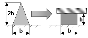
Abb. 1: Empfohlene Raupengeometrie
